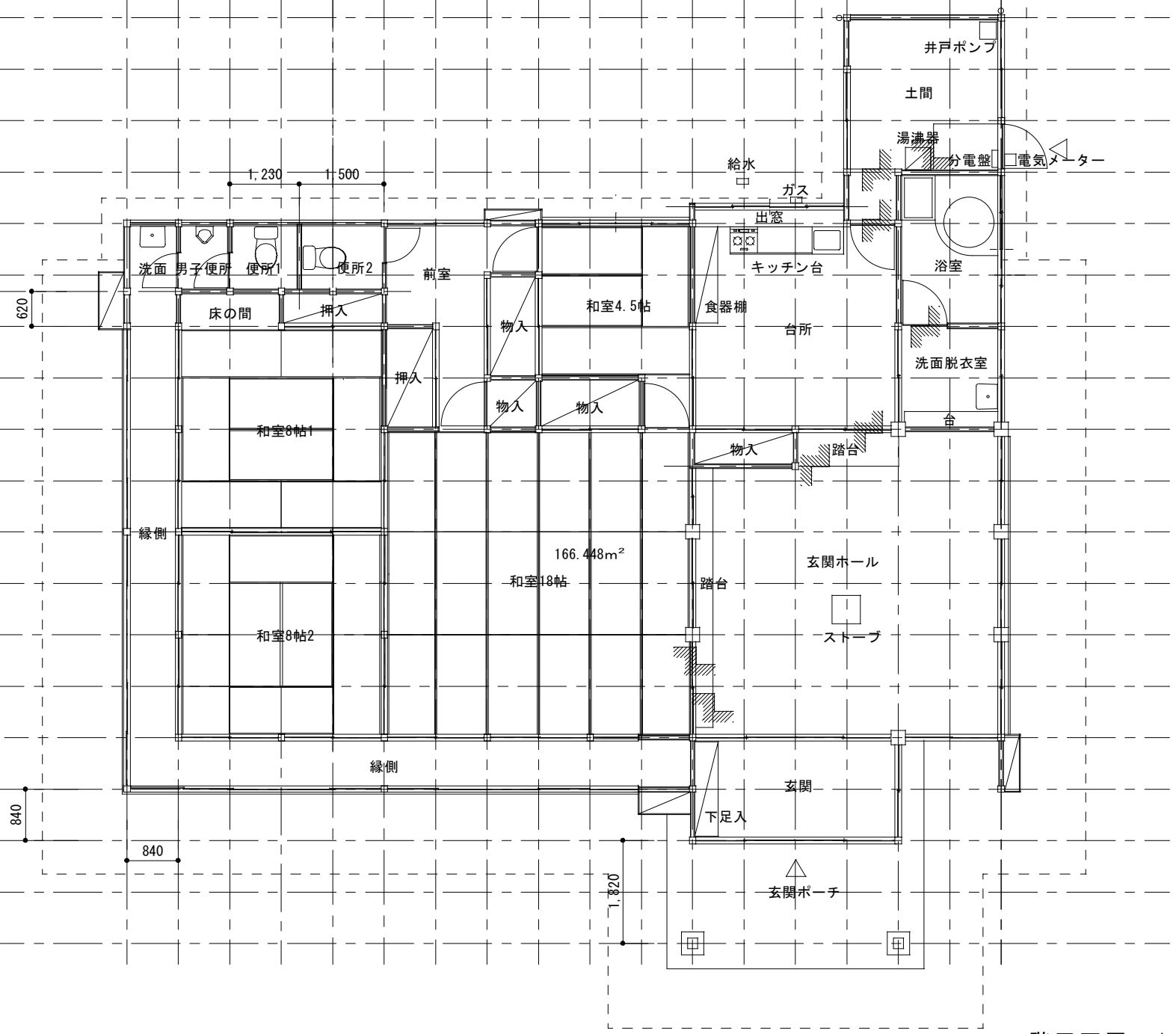
1階平面図 1:100
